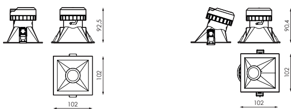
SOURCE LUMINEUSE + ACCESSOIRE SQ 60° SYMÉTRIQUE
