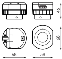
SOURCE LUMINEUSE
