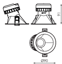
MOTOR LIGEIRO + ACESSÓRIO CL ASSIMÉTRICO 60°
