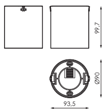
MOTOR LUMÍNICO + ACCESÓRIO SUPERFICIE
