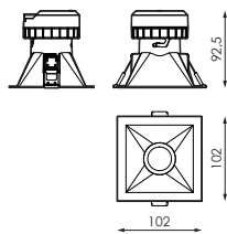
MOTOR LUMÍNICO + ACCESÓRIO SQ 60° SIMÉTRICO
