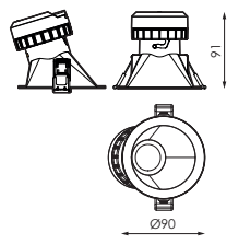
MOTOR LUMÍNICO + ACCESÓRIO CL 60°ASIMÉTRICO
