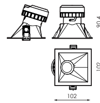
MOTOR LUMÍNICO + ACCESÓRIO SQ 60° ASIMÉTRICO
